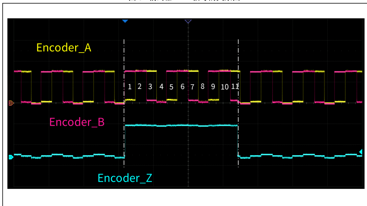
图 6. 编码器 ABZ 信号的关系图
