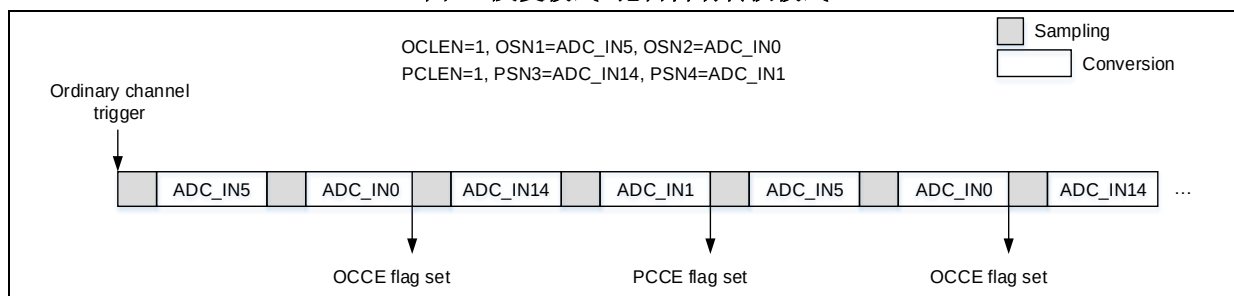
图 3. 反复模式+抢占自动转换模式
