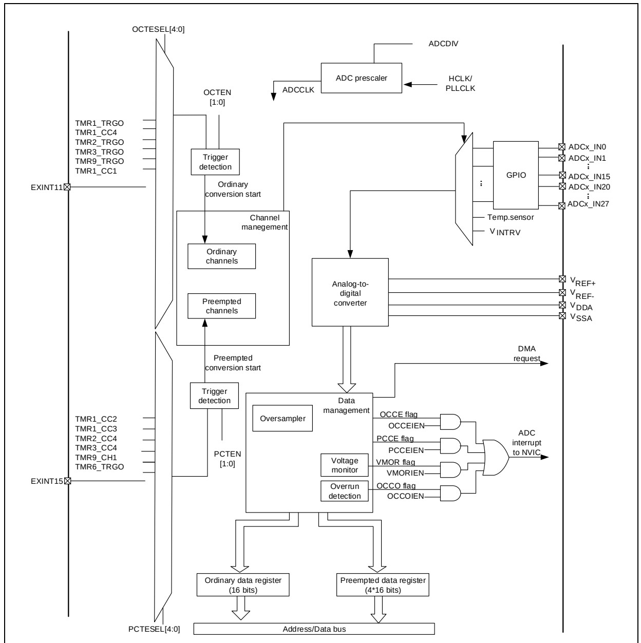
图 1. ADC1 框图
