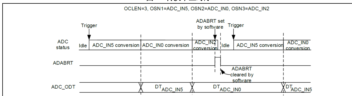
图 7. 转换中止时序
