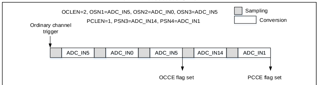
图 5. 抢占自动转换模式
