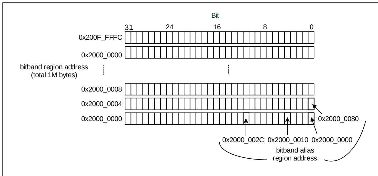
图 3.位带区与位带别名区的膨胀关系图 B
