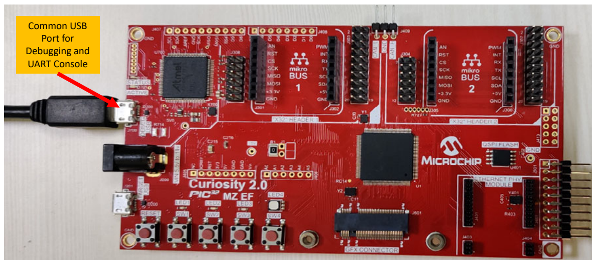
图 1-24. 硬件连接
