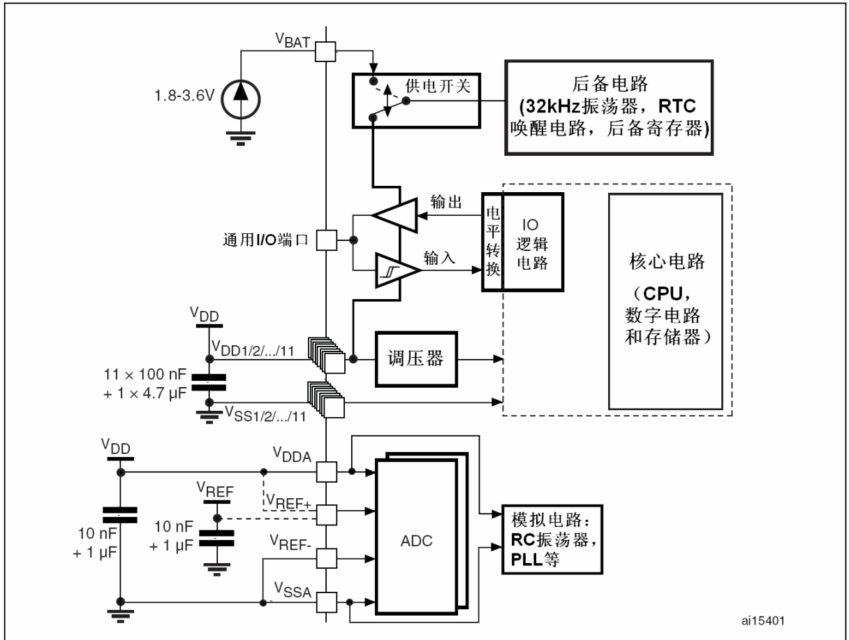
图9 供电方案
