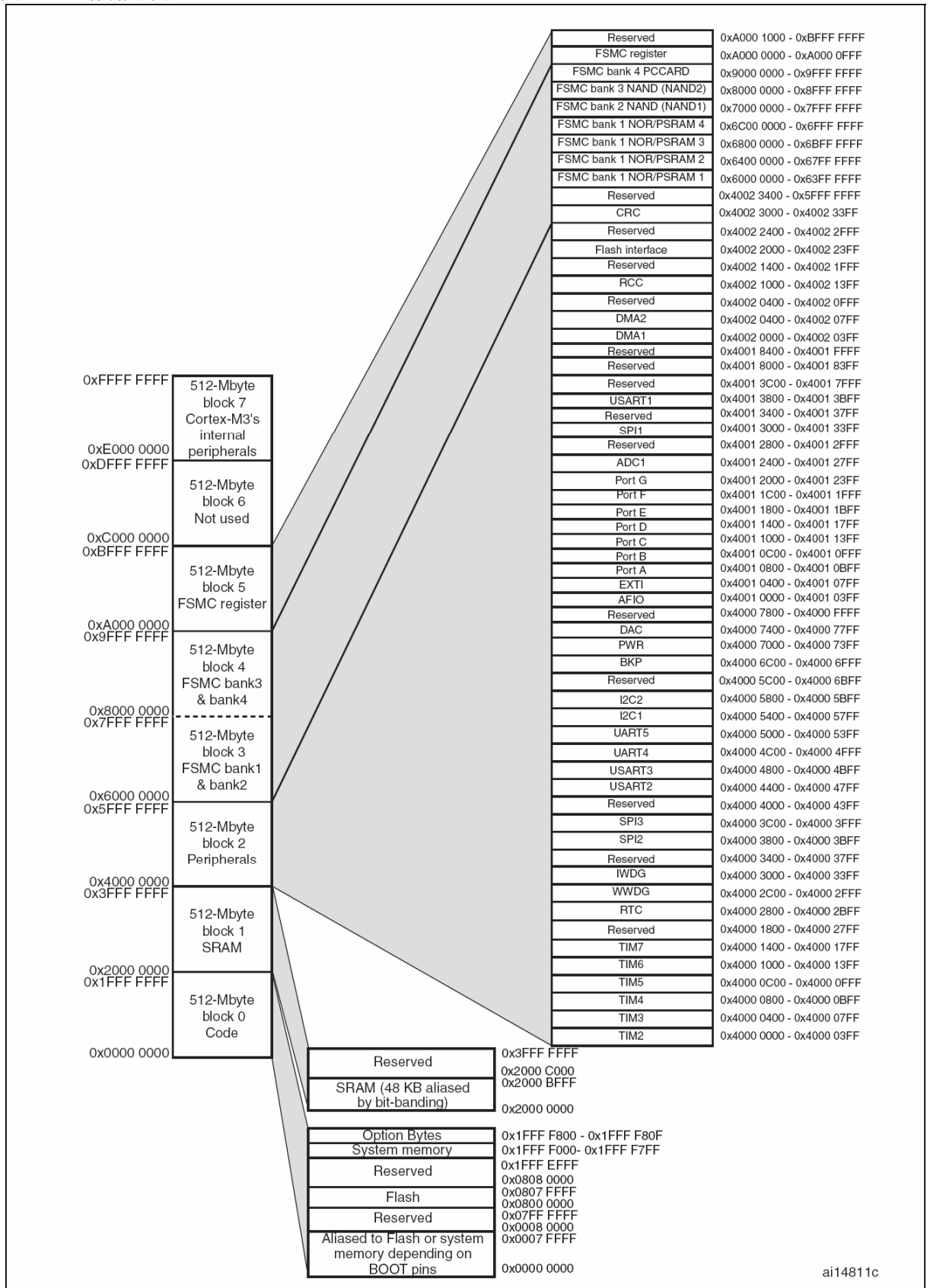
图6 存储器图
