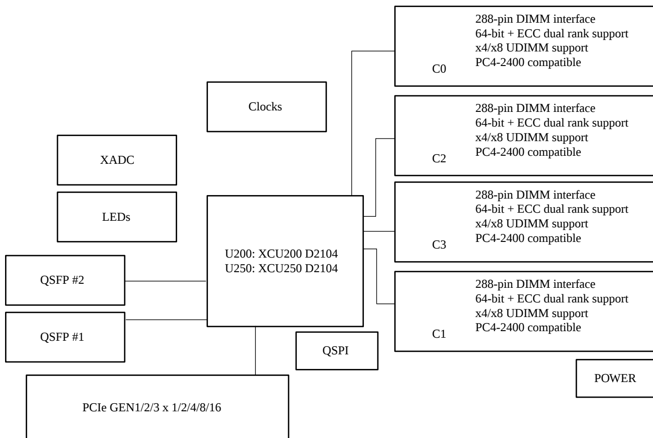
图 2: 卡原理图
