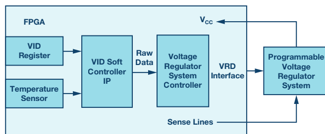
图4. Altera SmartVID结构。
