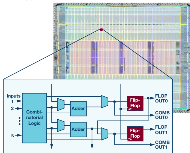
图25. FPGA可配置架构。
