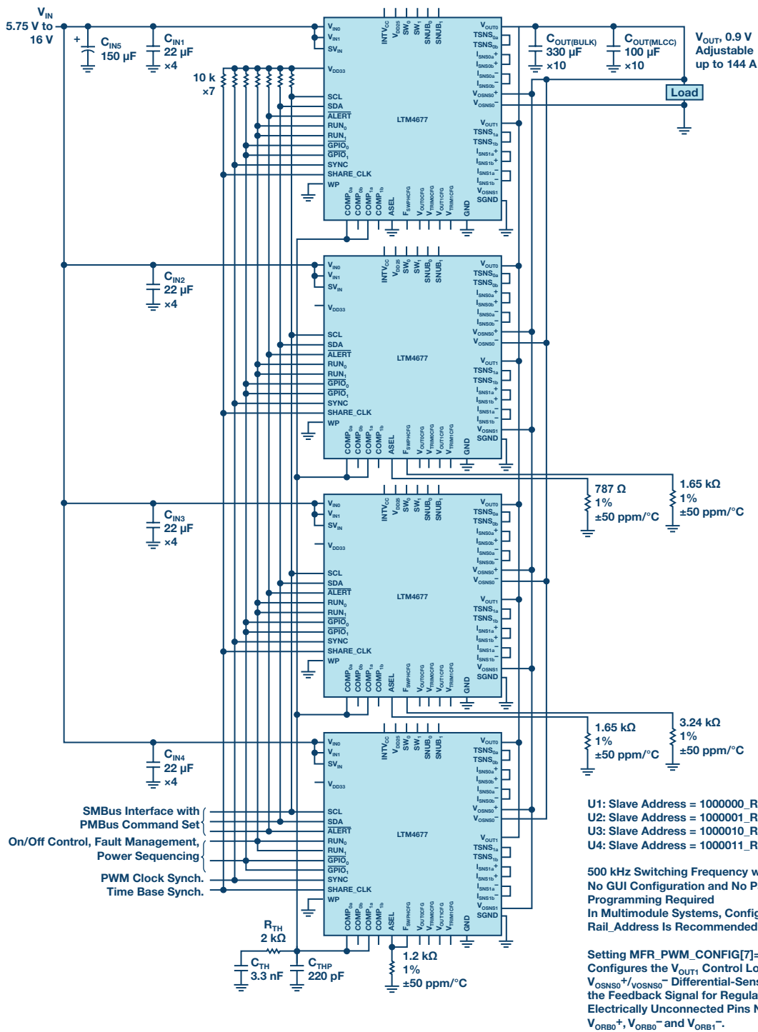
图19. 四个LTM4677在0.9 V下提供高达144 A的电流。
