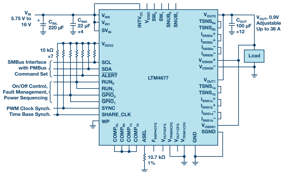
图18. 单个LTM4677提供高达36 A的电流。
