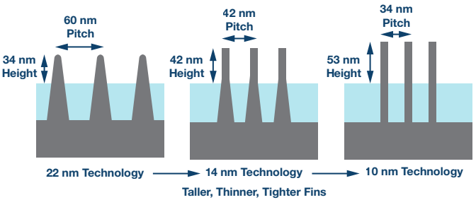
图22. 不断缩小的晶体管尺寸。
