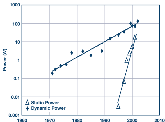
图23. 静态和动态功率增长率 9 。
