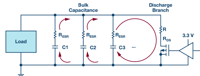
图13. 用FET对电源电容放电。
