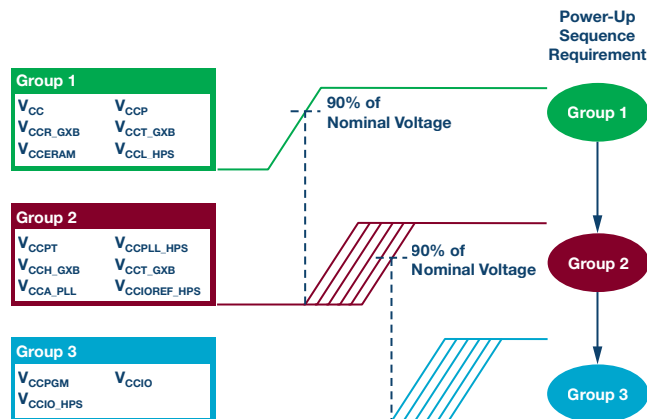
图6. Altera Arria 10升序序列组。
