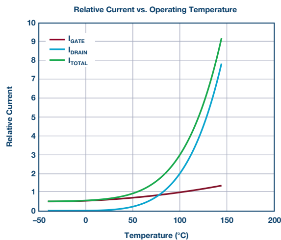
图3. 电源电流与工作温度的关系。
