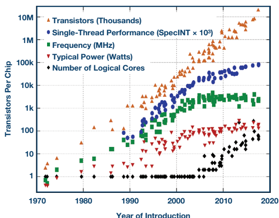
图24. 计算硬件指标的增长趋势。
