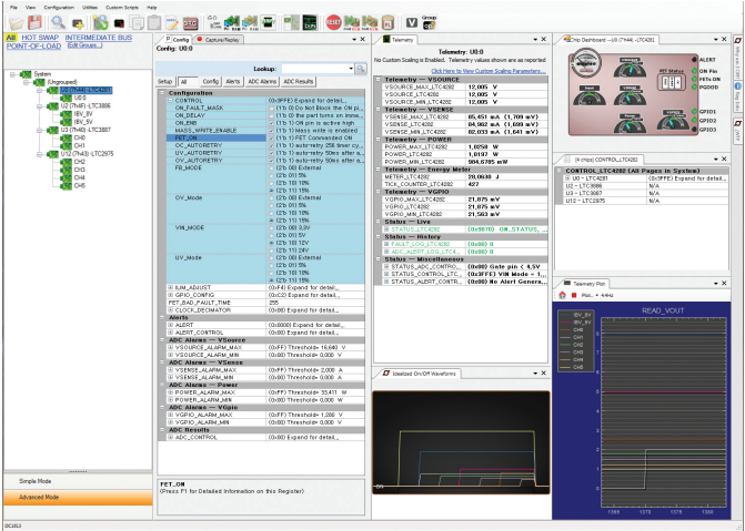
图21. LTpowerPlay图形用户界面。
