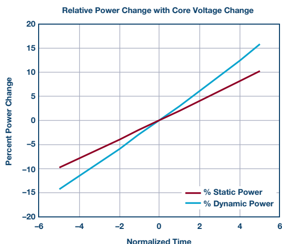
图1. Xilinx Virtex V功率与内核V CC 。
