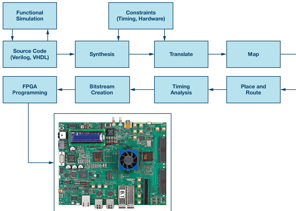
图27. FPGA设计流程（硬件最后）。
