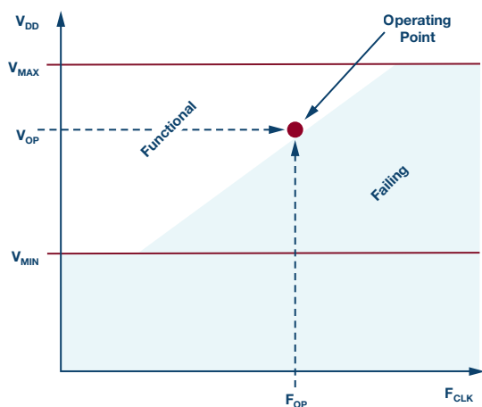
图5. FPGA工作频率与 V_{DD} 之间的平衡关系。
