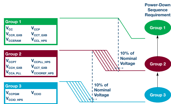
图12. Altera Arria 10降序序列组。
