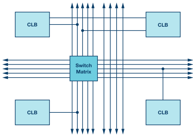
图26. CLB之间可配置的开关矩阵。
