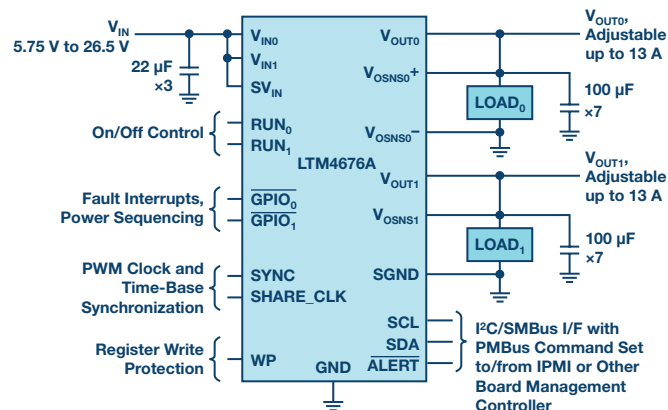
图11. LTM4676A PSM μ模块双通道13 A调节器。
