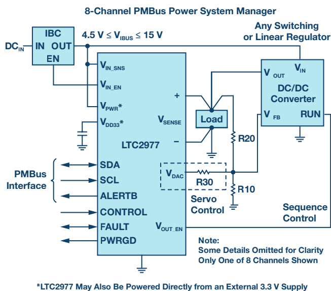
图20. LTC2977可管理任意电源电压。
