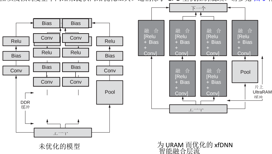
图 9: xFDNN 编译器优化
