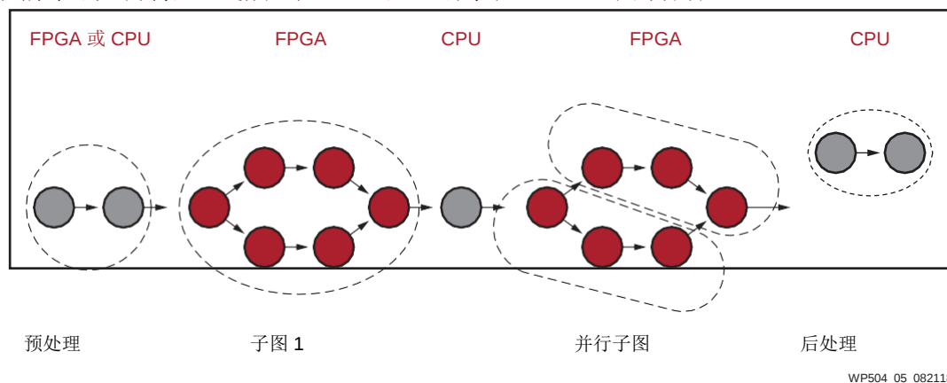
图 5: 由编译器分区处理
