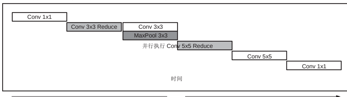
图 3: GoogLeNet v1 中 Inception 层的 xDNN 调度
