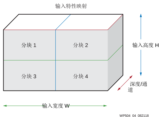
图 4: 硬件辅助图像分块功能
