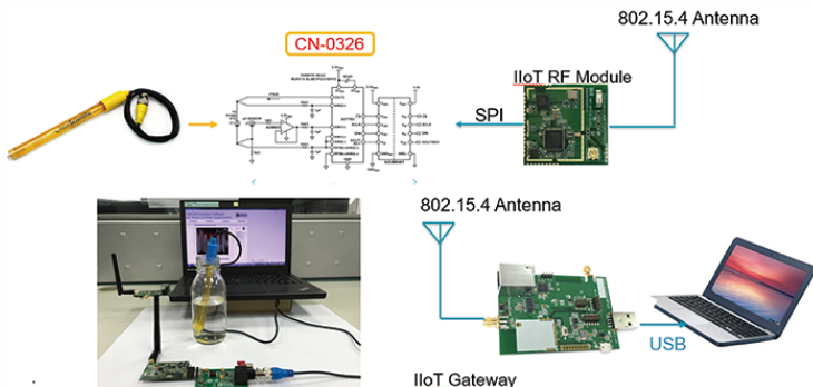
Fig.2 OPR sensor + CN0326+ IIoT Module
