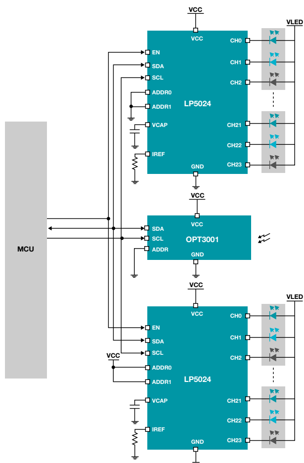
图 6. 各种 LED 环形灯照明图案参考设计
